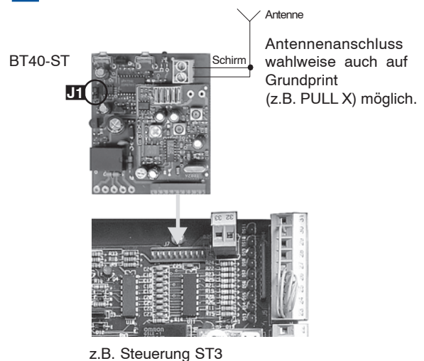
z.B. Steuerung ST3
