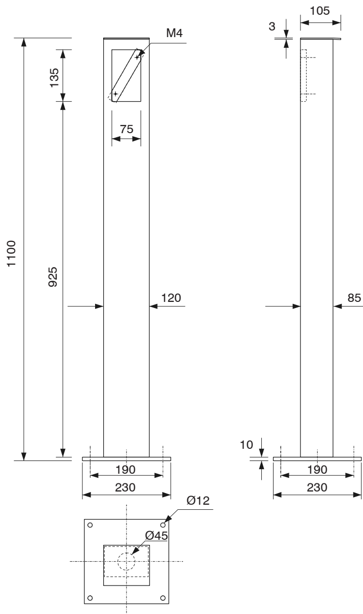
Maßskizze GSB Säule für PKW (Maße in mm)
